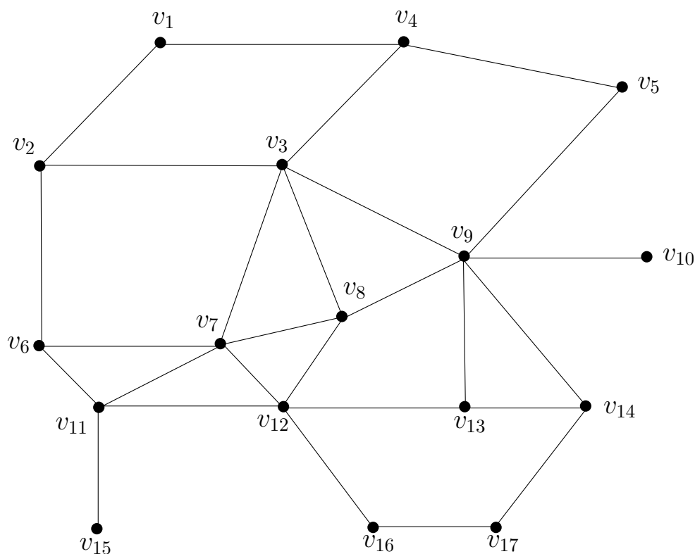
Abbildung 1: Der Graph G .
