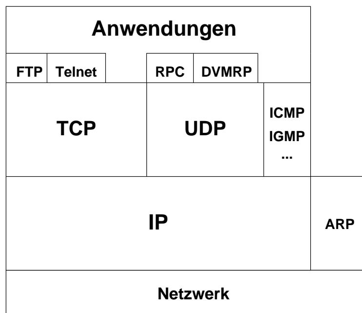
Abbildung 1: Internet-Protokolle
