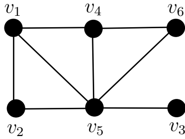
Abbildung 1: Der Graph H .
