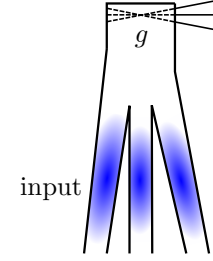
(d) And gadget.
