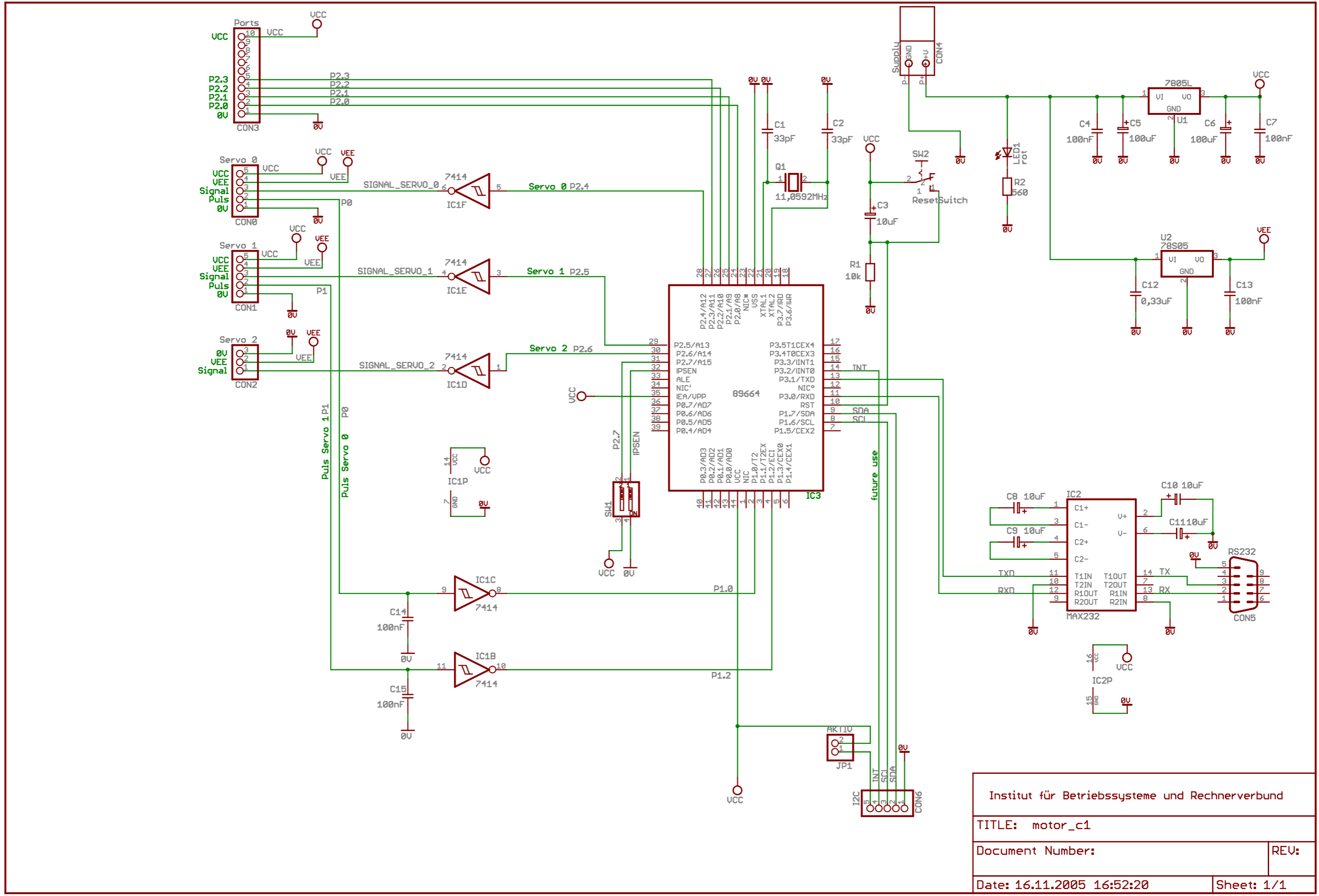
Abbildung B.5: Schaltbild
