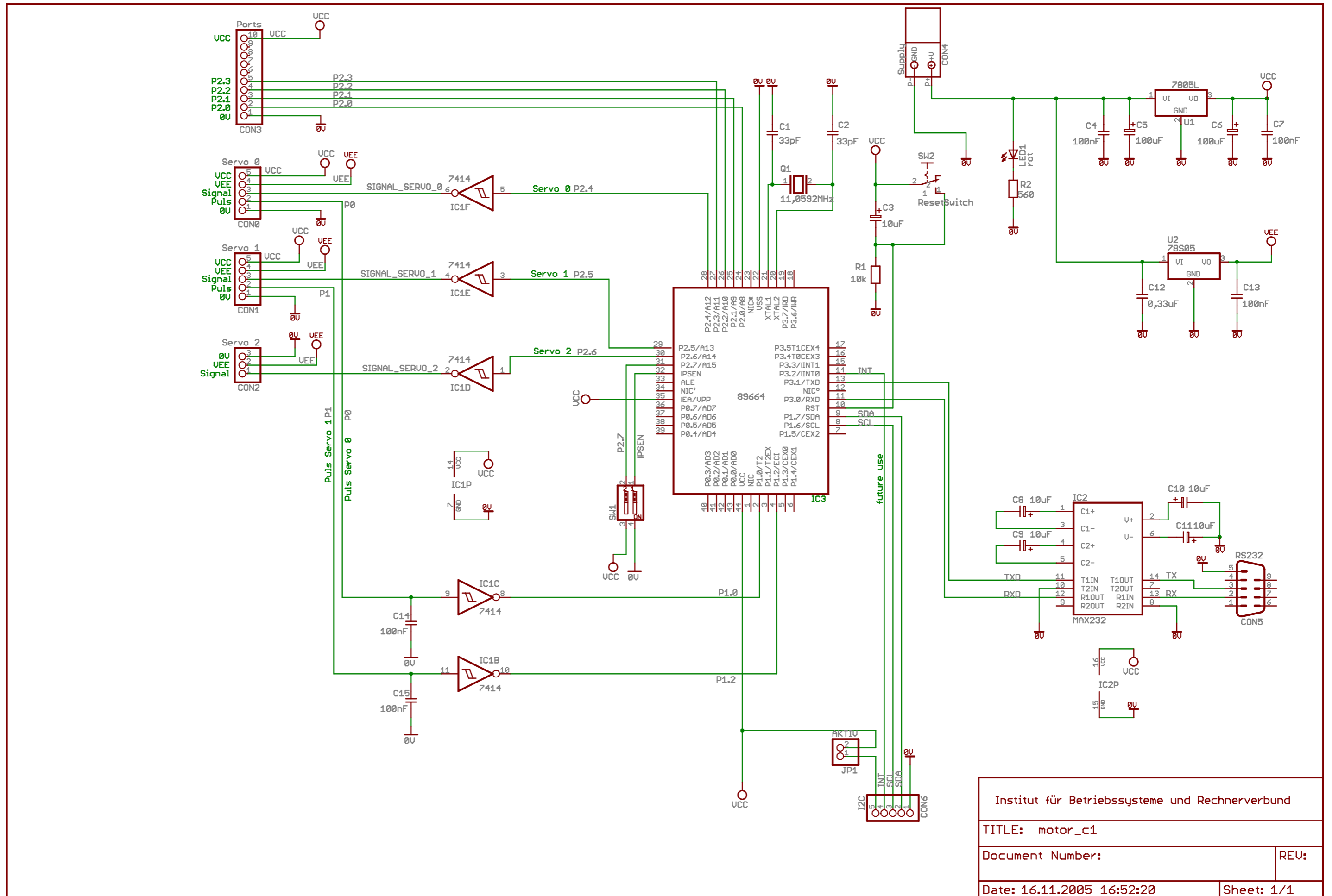
Abbildung 7.5: Schaltbild
